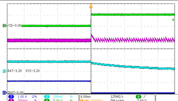
图 9-3. 断电
