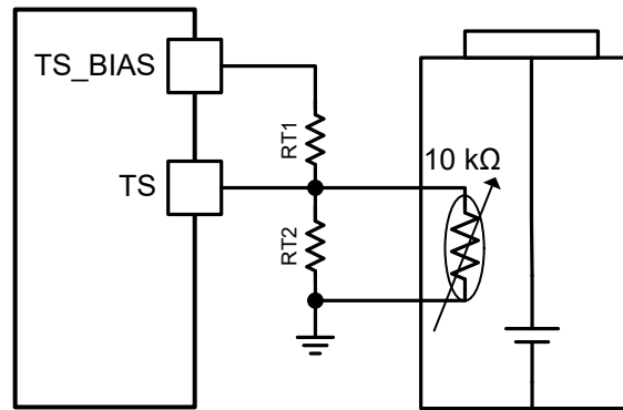
图 8-3. TS 电阻器网络
