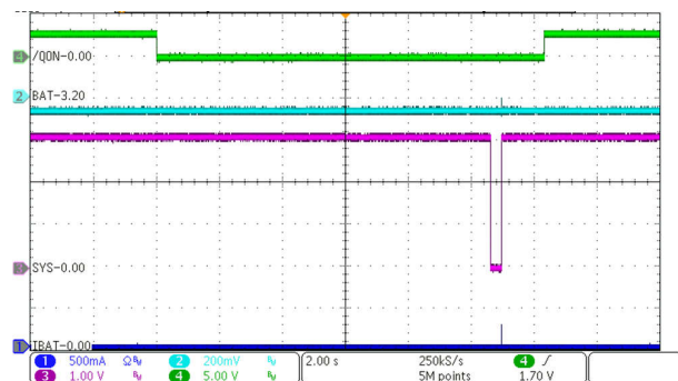
图 9-4. 充电启用
