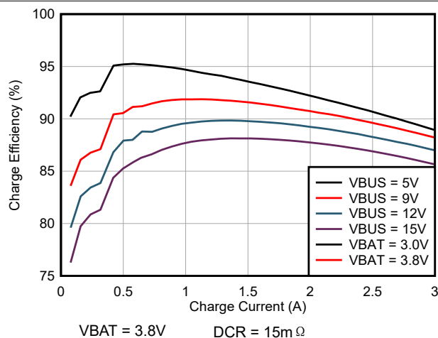
图 7-1. 充电效率与充电电流间的关系
