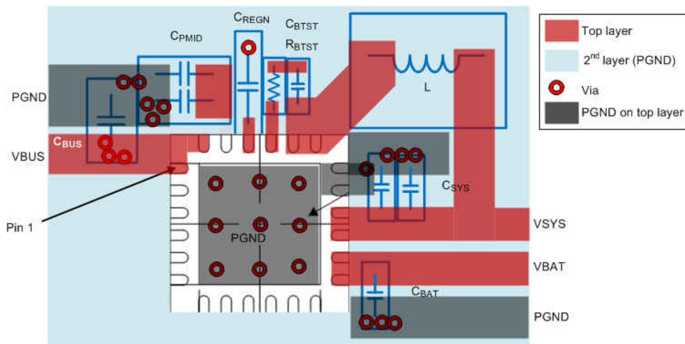
图 12-2. Layout Example
