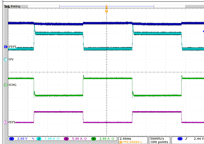
图 10-14. OTG Switching
