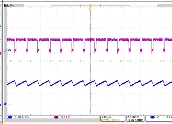
图 10-7. PFM Switching in Buck Mode
