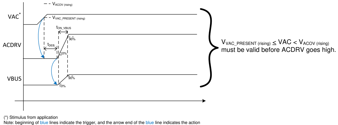
图 9-1. ACFET Startup Control
