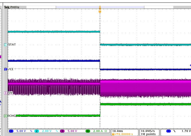
图 10-11. Charge Enable
