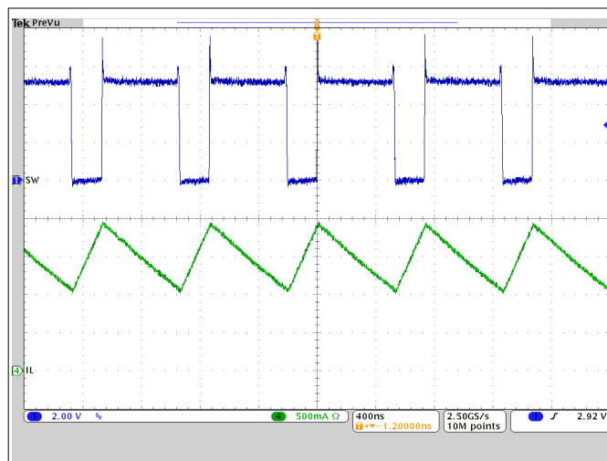
图 10-14. OTG Switching
