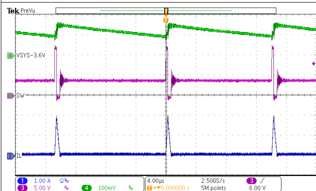
图 10-4. PFM Switching in Buck Mode
