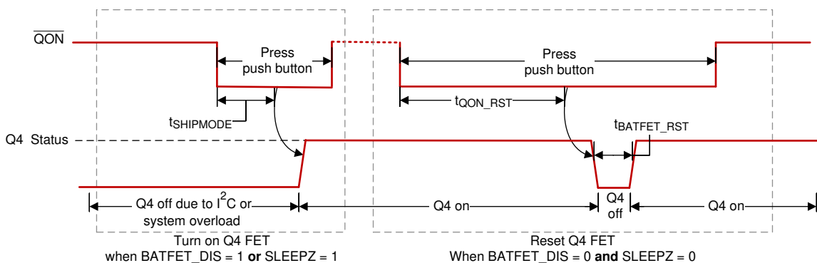
图 8-10. QON Timing
