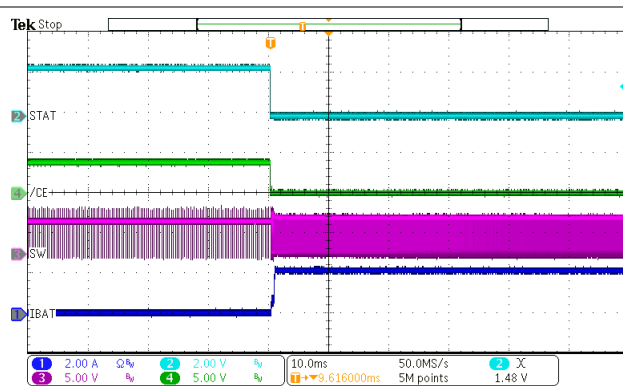
图 9-10. Charge Enable
