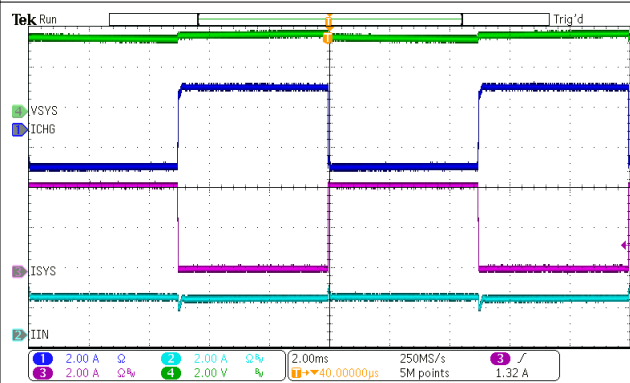
图 9-18. System Load Transient
