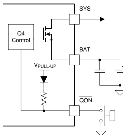
图 8-11. QON Circuit
