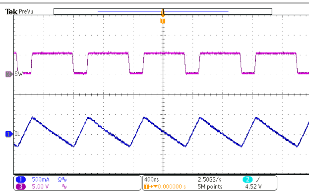
图 9-12. OTG Switching
