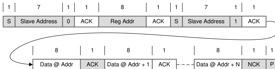
图 8-19. Multi-Read
