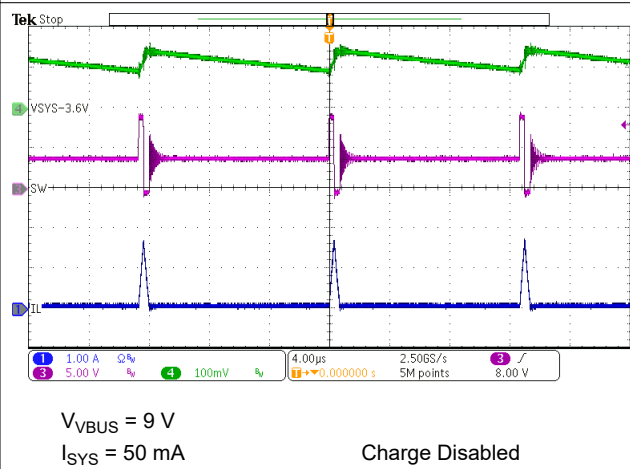
图 9-6. PFM Switching in Buck Mode
