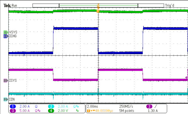
图 9-16. System Load Transient
