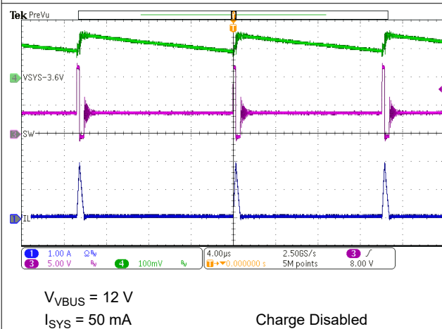
图 9-7. PFM Switching in Buck Mode
