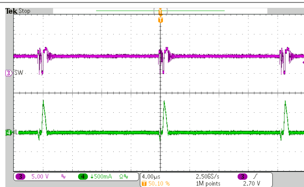
图 9-10. Charge Enable
