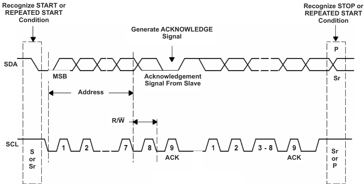
图 6-12. 总线协议
