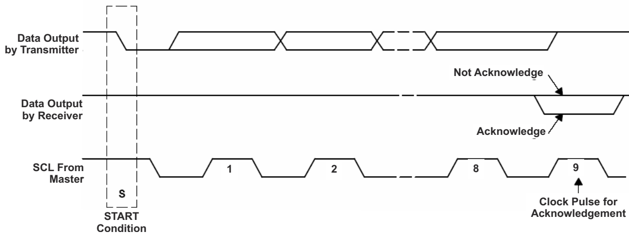
图 6-11. I 2 C 总线上的确认
