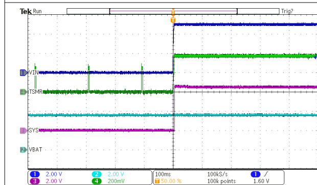
图 7-2. 在没有电池的情况下通过插入 IN 电源进行上电
