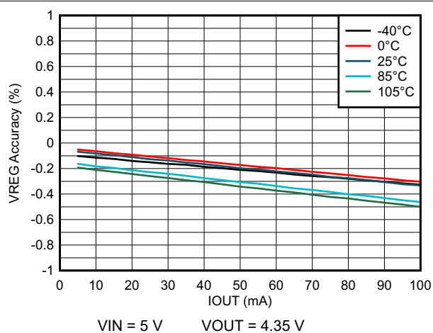
图 6-2. Load Regulation
