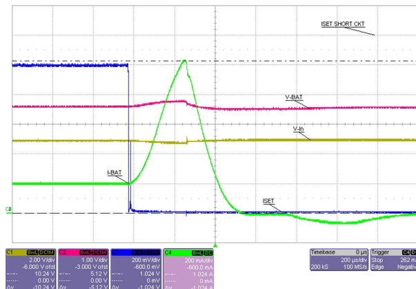
图 8-9. ISET Short-Circuit Response
