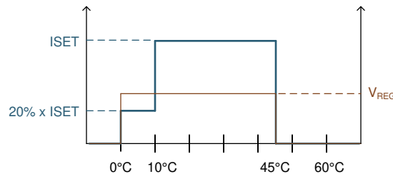
图 7-3. BQ25175 Charging Profile
