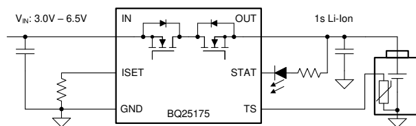
简化版原理图
