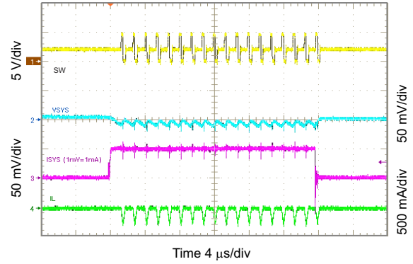
图 10-33. 2.1 V_{SYS} Load Transient, 0 to 50 mA
