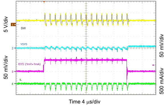
图 10-32. 1.8 V_{SYS} Load Transient, 0 to 50 mA
