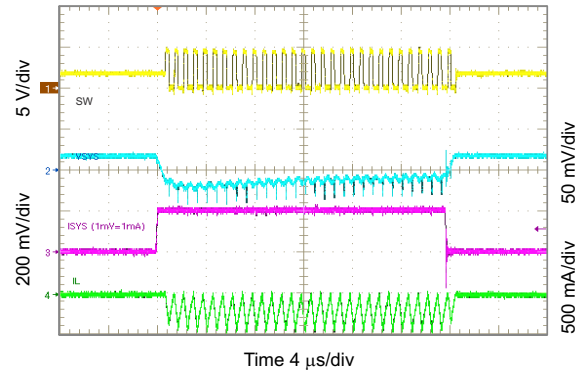
图 10-35. 3.3 V_{SYS} Load Transient, 0 to 50 mA
