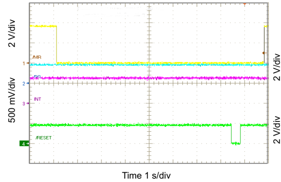
图 10-64. RESET Timing
