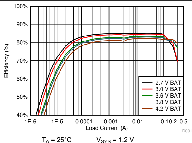
图 10-8. 1.2 V_{\text{SYS}} System Efficiency
