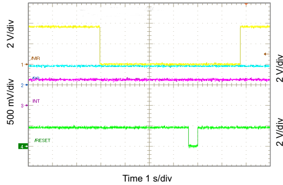
图 10-63. RESET Timing
