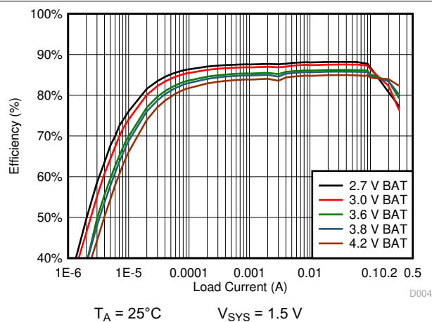
图 10-9. 1.5 V_{\text{SYS}} System Efficiency
