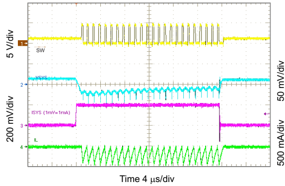
图 10-34. 2.5 V_{SYS} Load Transient, 0 to 50 mA
