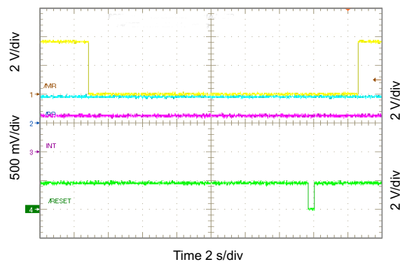
图 10-63. RESET Timing
