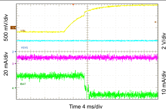
图 10-7. OVP Fault
