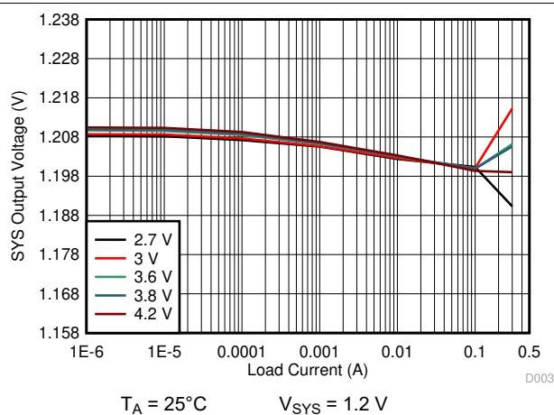
图 10-13. 1.2 V_{\text{SYS}} Load Regulation
