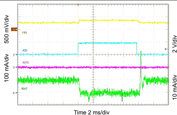
图 10-6. Charger On/Off Using \overline{CD}
