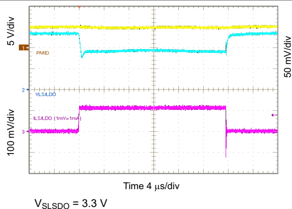
图 10-56. 3.3 V_{LSLDO} Load Transient, 0 to 100 mA
