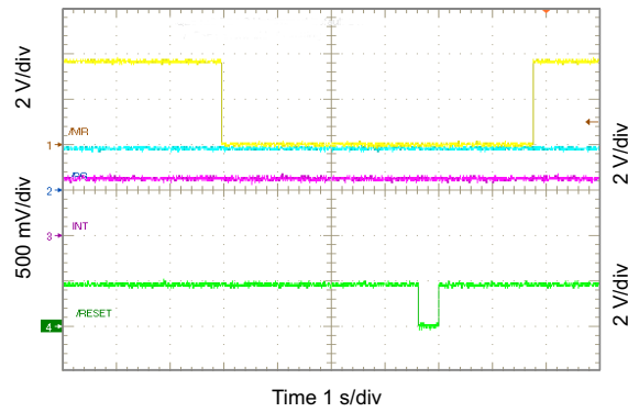
图 10-65. RESET Timing
