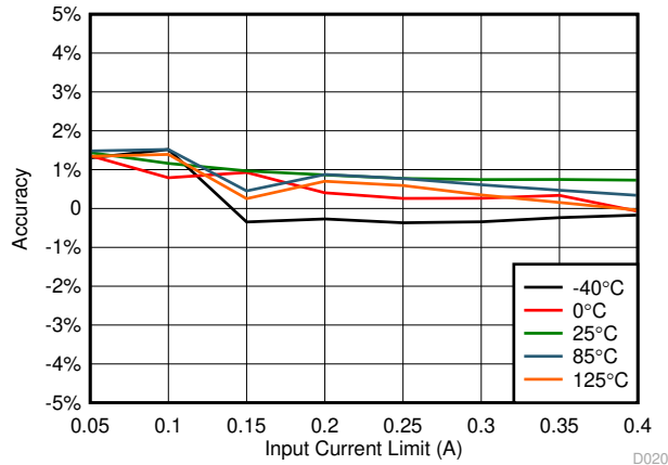
图 8-9. ILIM Accuracy vs Input Current
