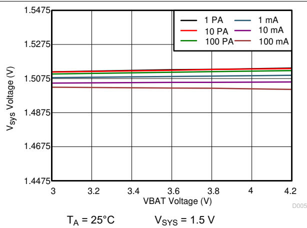
图 10-21. 1.5 V_{SYS} Line Regulation
