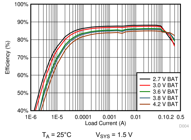
图 10-11. 1.5 V_{\text{SYS}} System Efficiency
