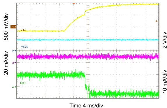
图 10-9. OVP Fault
