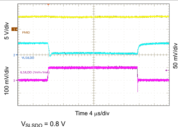
图 10-52. 0.8 V_{LSLDO} Load Transient, 0 to 100 mA
