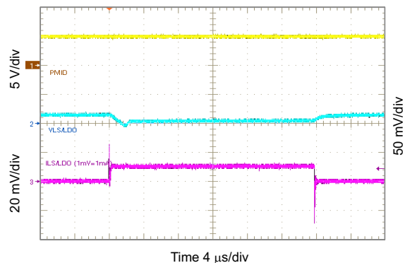
图 10-47. 0.8 V_{LSLDO} Load Transient, 0 to 10 mA
