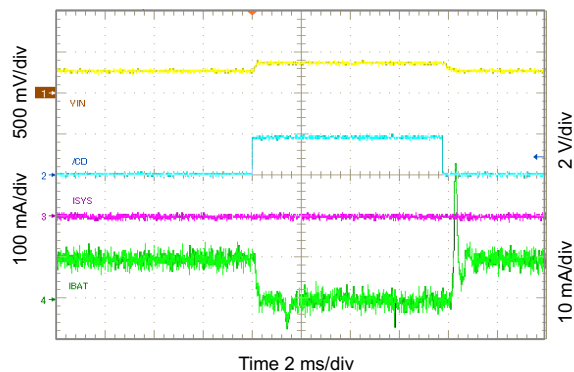
图 10-8. Charger On/Off Using \overline{CD}
