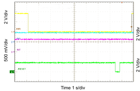
图 10-66. RESET Timing
