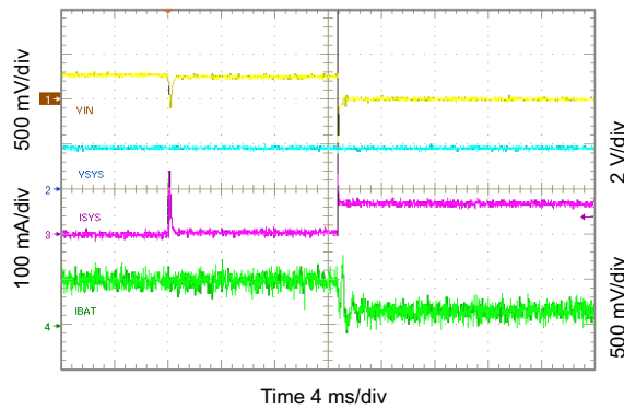
图 10-4. Entering DPPM Mode
