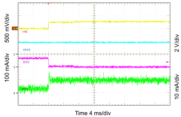
图 10-5. Exiting DPPM Mode
