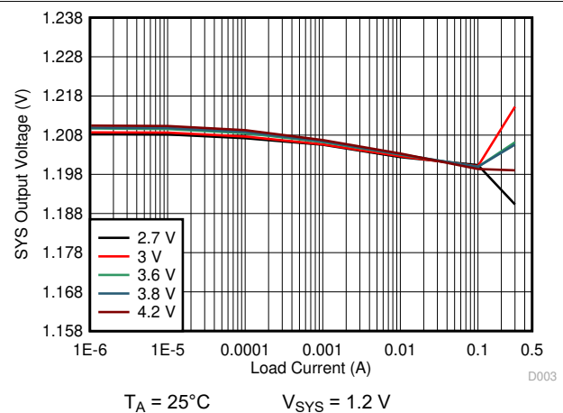
图 10-15. 1.2 V_{\text{SYS}} Load Regulation
