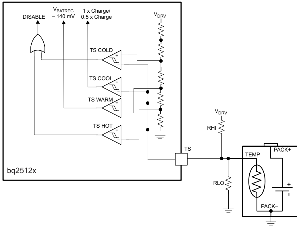
图 16. TS Circuit
