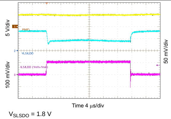
图 88. 1.8 V_{SLSDO} Load Transient, 0 to 100 mA
