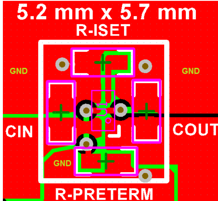
图 28. Board Layout
