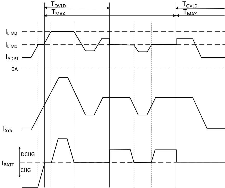
图 6-2. 两级适配器电流限制时序图, REG0x37[8] = 0
