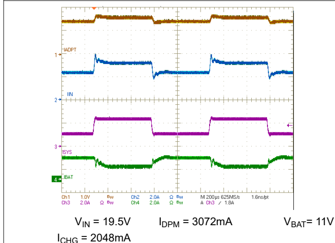
V_{IN} = 19.5V I_{DPM} = 3072mA V_{BAT} = 11V I_{CHG} = 2048mA 图 7-14. 系统负载瞬态期间的输入电流调节
