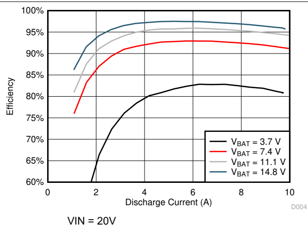
图 5-5. 混合升压期间的效率
