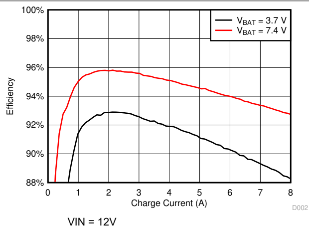
图 5-3. 充电期间的效率
