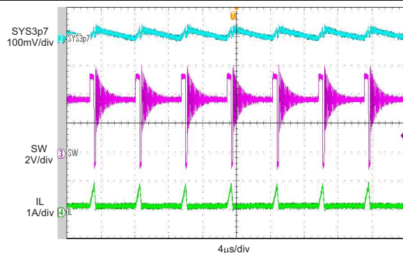
图 41. Charge Disable
