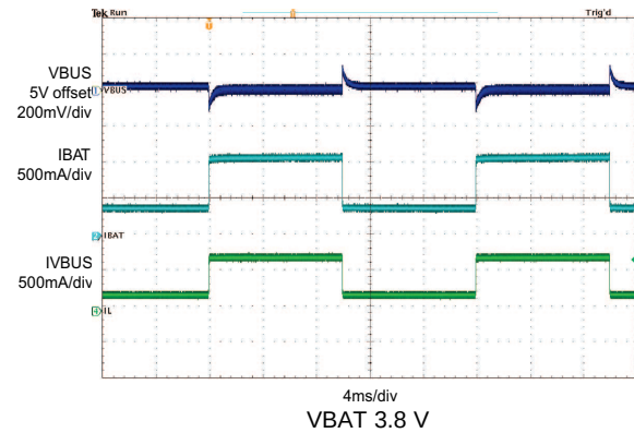
图 47. Boost Mode Enable
