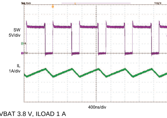
图 46. PFM Switching Waveform
