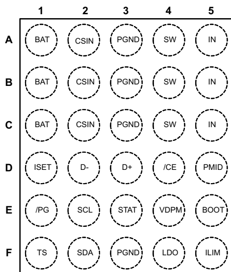
bq24257 WCSP
