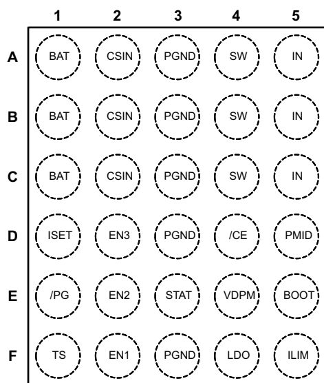
bq24258 WCSP
