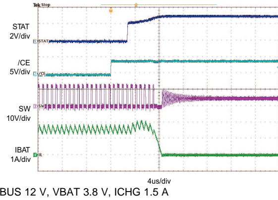
图 44. PWM Switching Waveform
