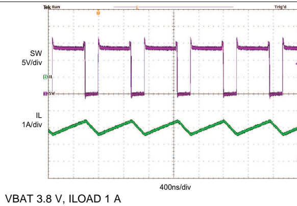
图 44. PWM Switching Waveform
