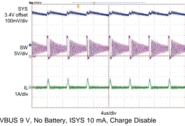
图 45. PFM Switching Waveform
