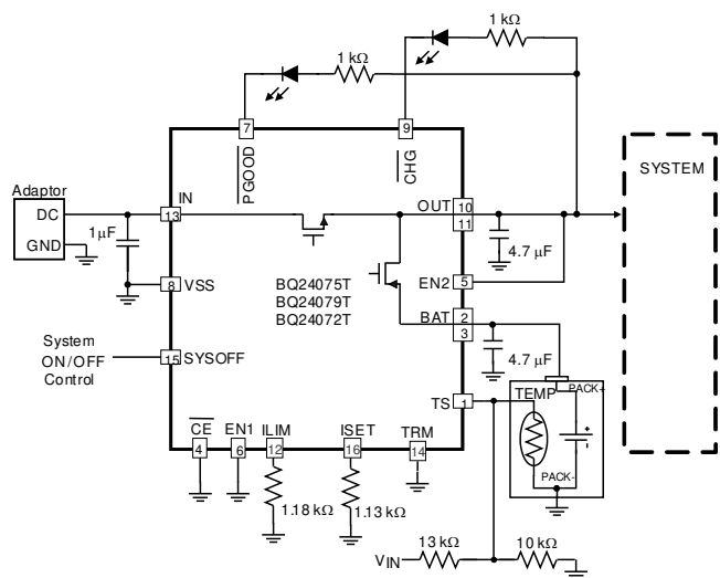
简化电路
