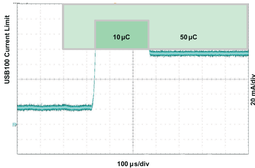
图 9-2. USB-IF Inrush Current Test
