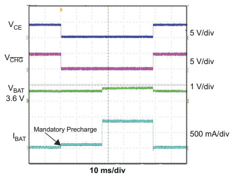
图 10-8. Charger ON/OFF Using \overline{\text{CE}}
