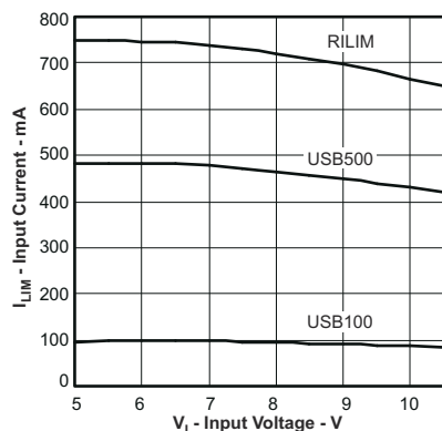
图 8-11. BQ24074 Input Current Limit vs Input Voltage
