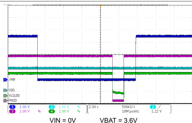
图 8-6. HW Reset on \overline{\text{MR}} Long Button Press
