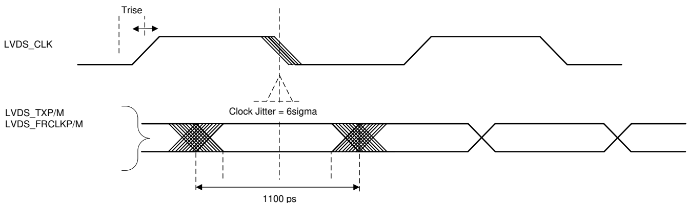
图 7-22. 计时参数
