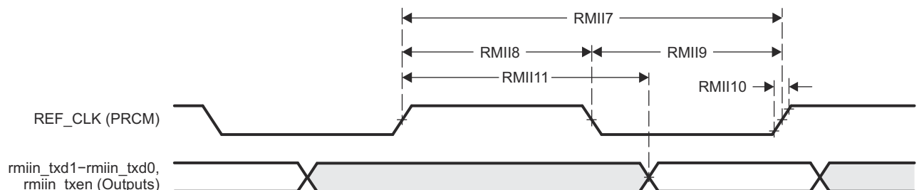
图 6-14. MAC 发送接口时序，RMII in 运行模式
