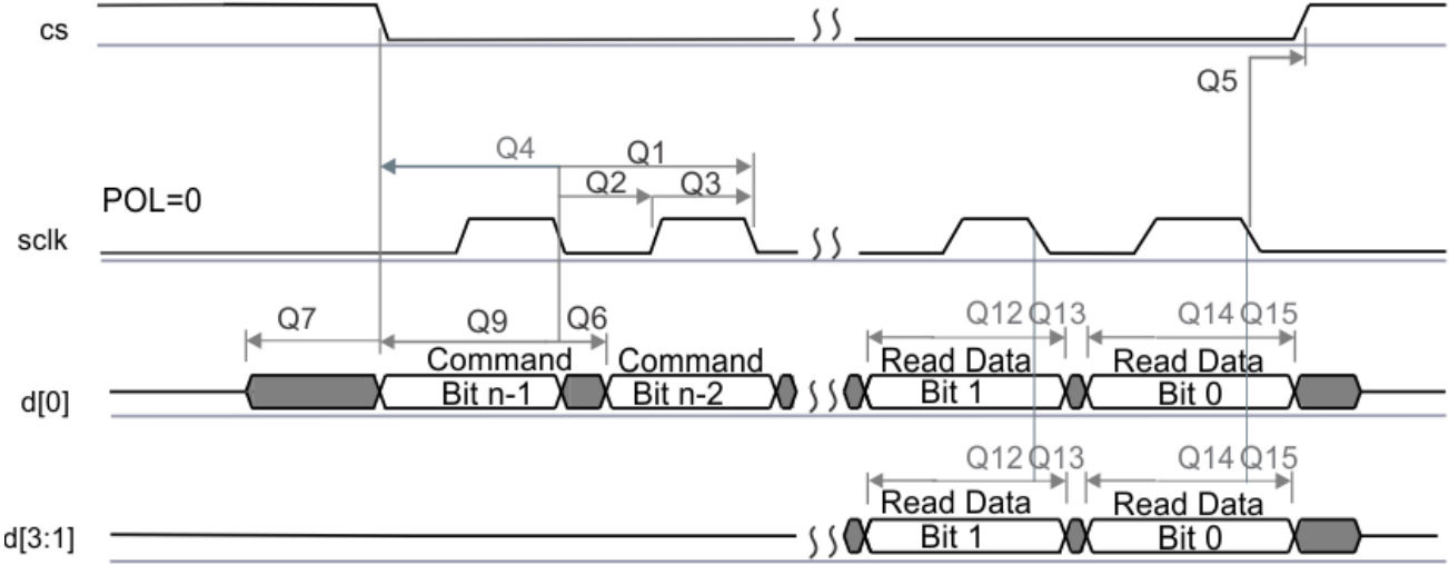
图 6-4. QSPI 读取 (时钟模式 0)
