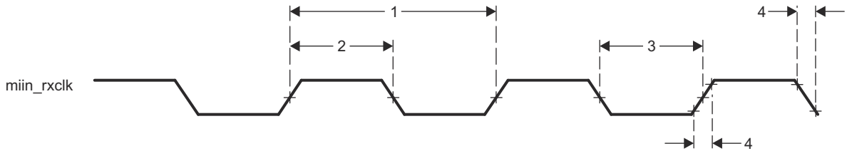
图 6-17. 时钟时序 (MAC 接收) — MIIn 运行模式
