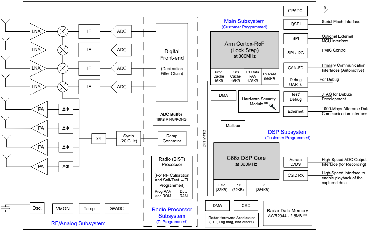
图 3-1. 功能方框图
