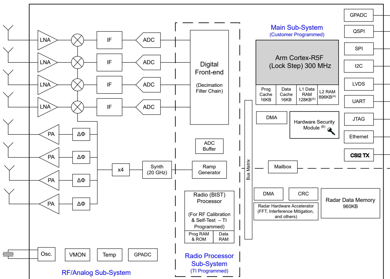
图 8-1. 功能方框图
