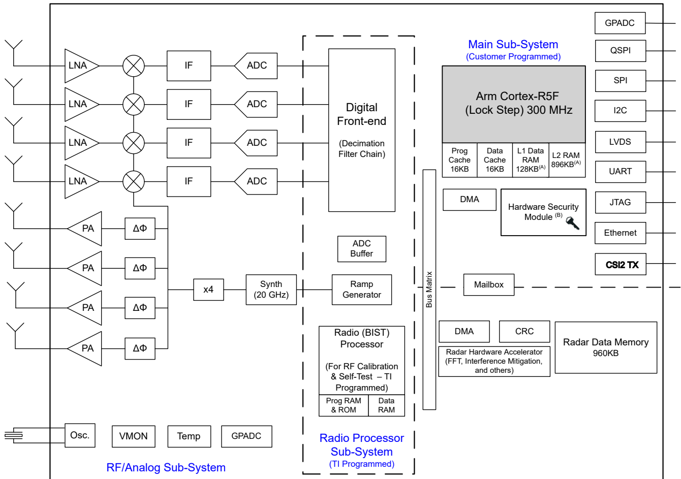
图 3-1. 功能方框图
