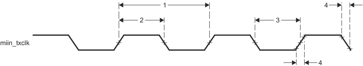
图 7-21. 时钟时序 (MAC 发送) - MIIn 运行模式
