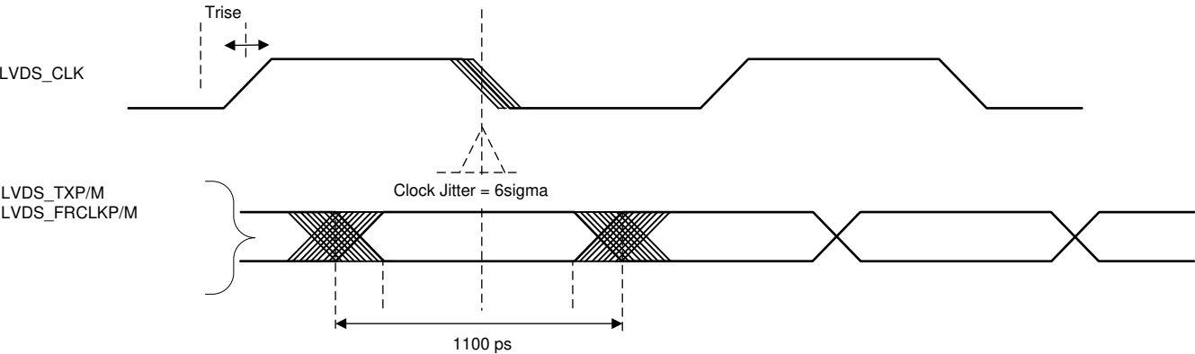
图 7-24. 计时参数
