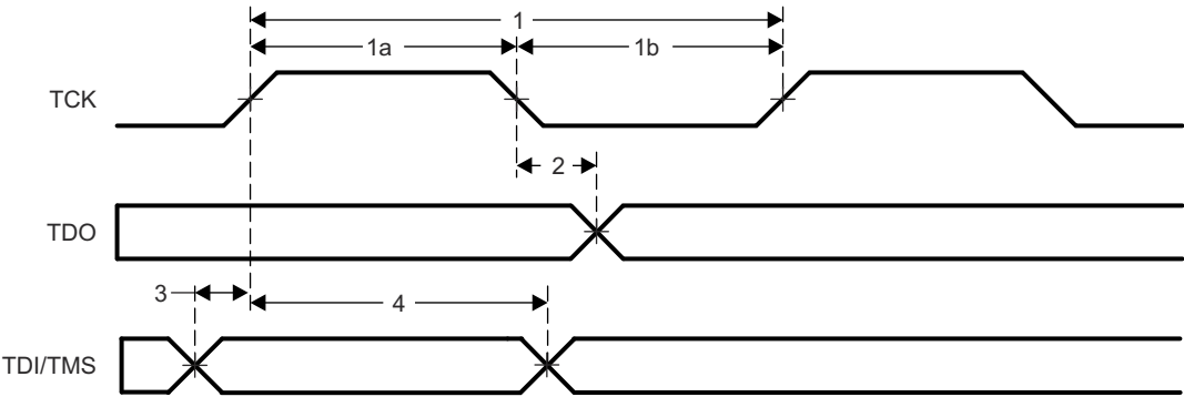
图 7-26. JTAG 时序
