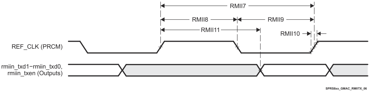
图 7-16. MAC 发送接口时序，RMII n 运行模式
