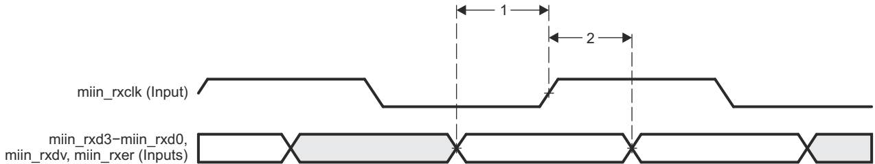
图 7-20. MAC 接收接口时序，MIIn 运行模式
