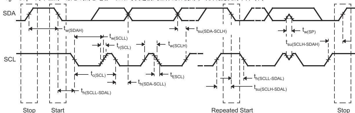
图 7-25. I2C 时序图
