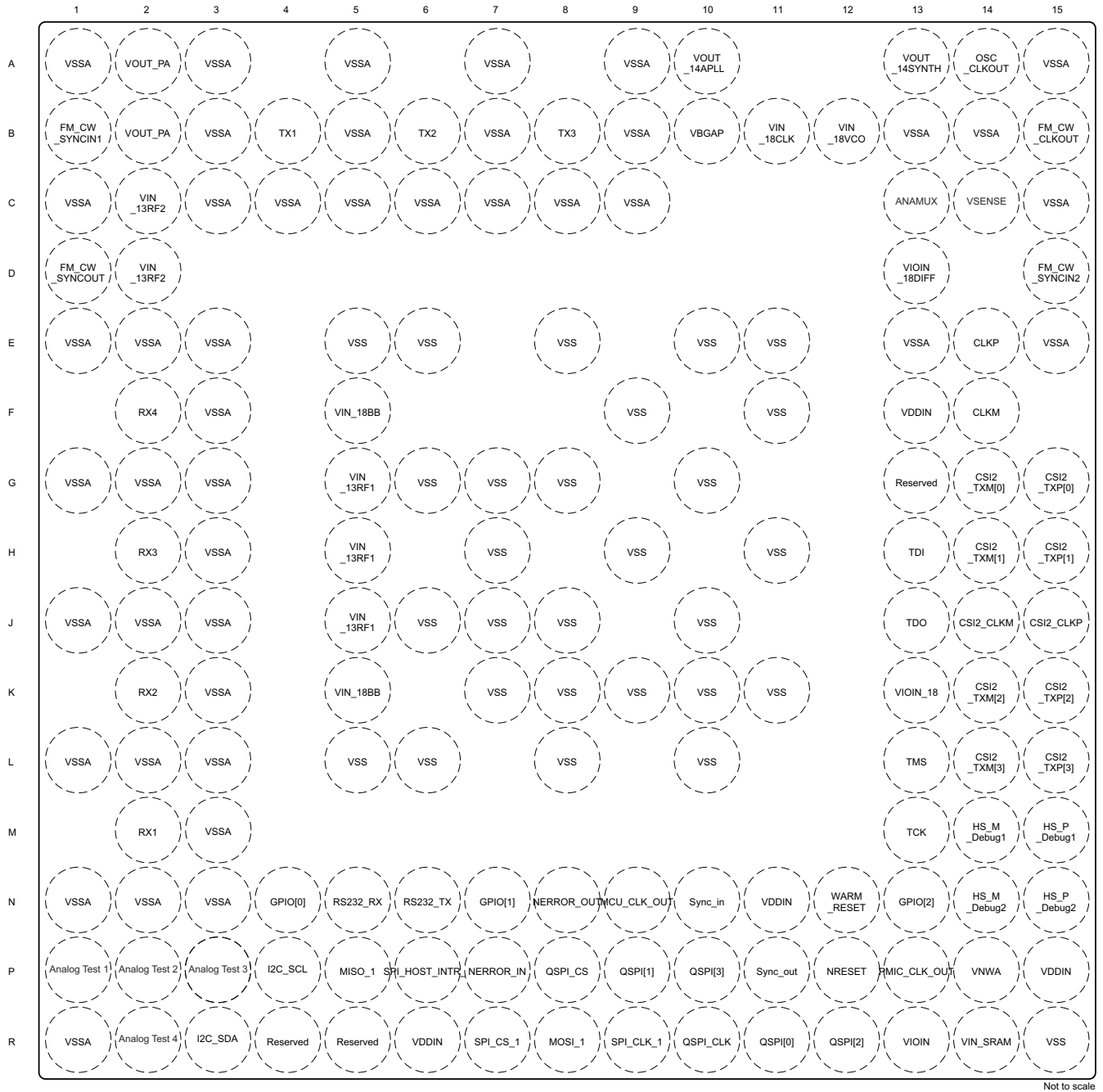
图 6-1. Pin Diagram
