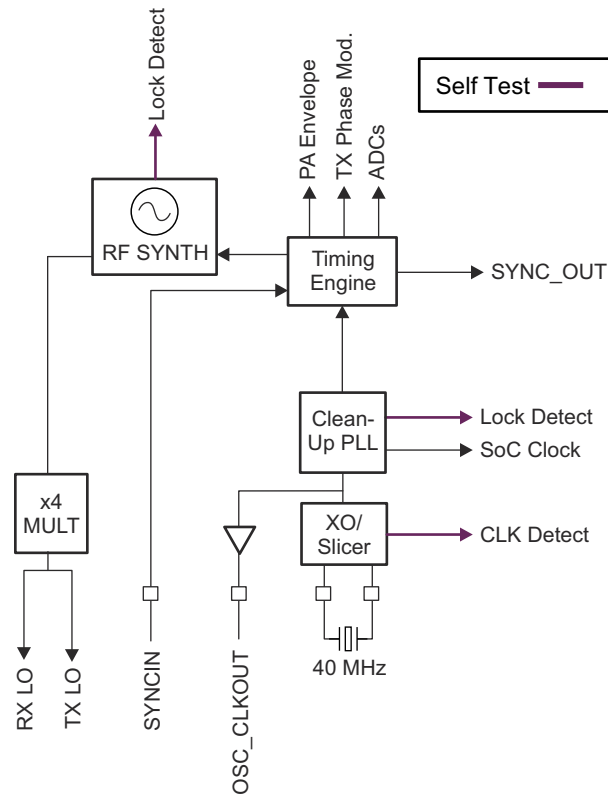
图 7-1. Clock Subsystem
