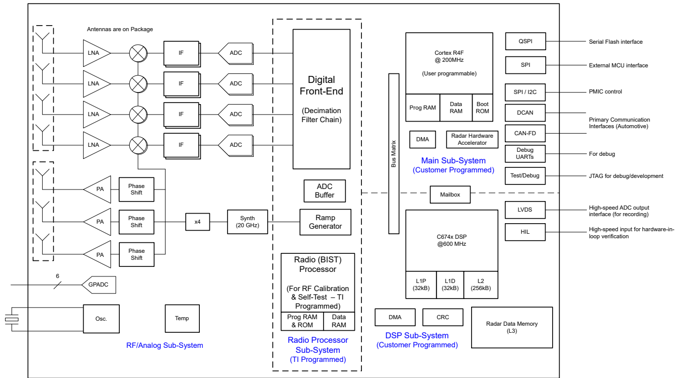
图 3-1. 功能方框图
