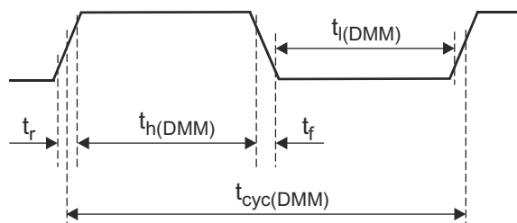
图 6-22. DMMCLK Timing
