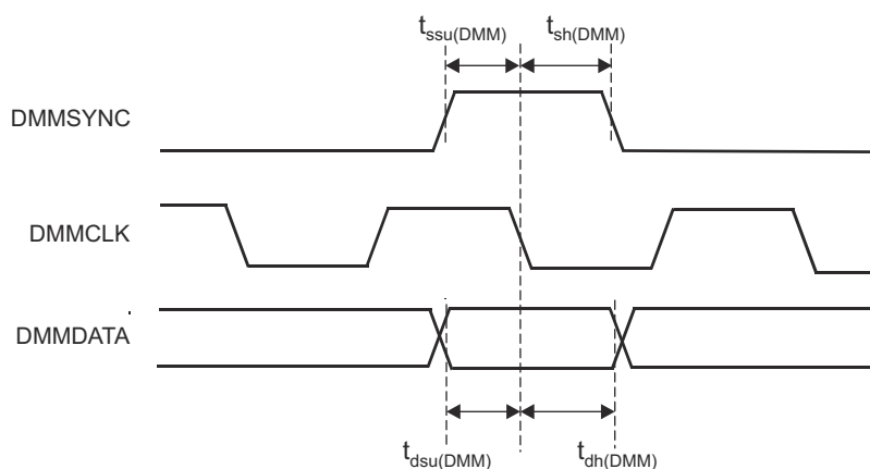
图 6-23. DMMDATA Timing
