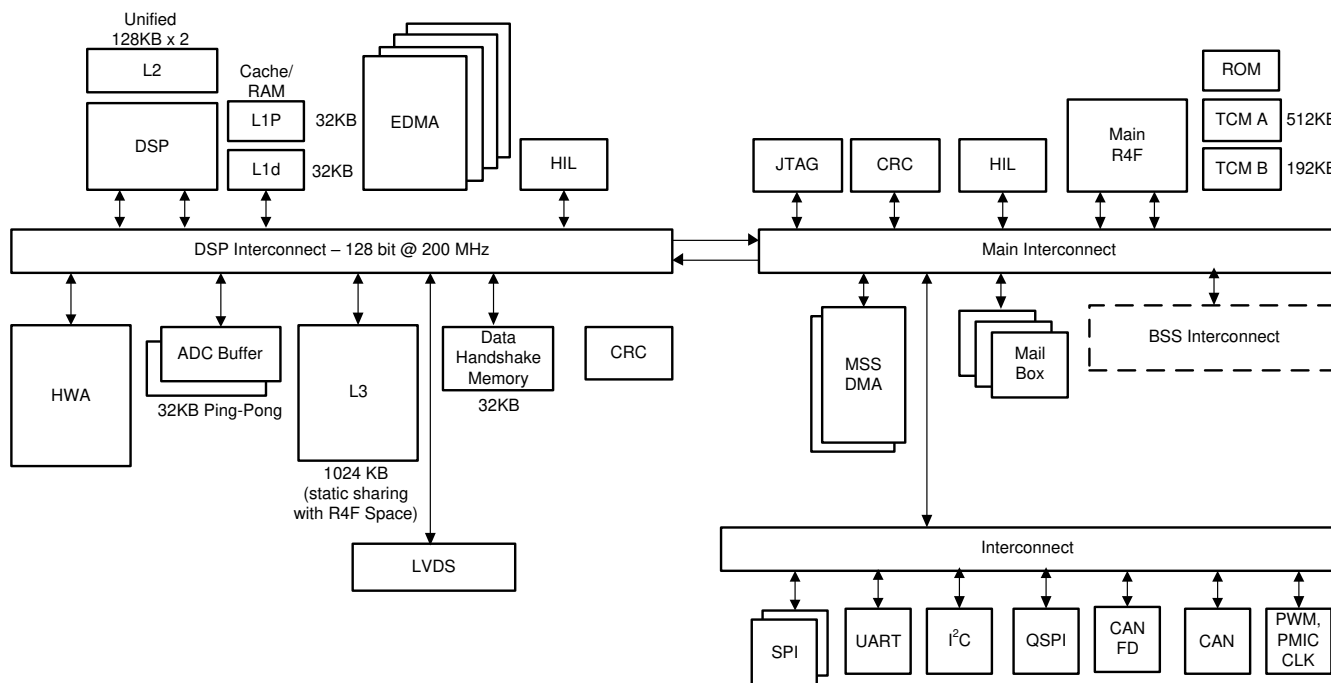
图 7-4. Processor Subsystem
