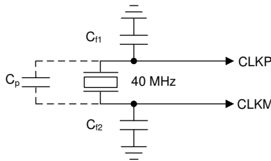
图 6-7. Crystal Implementation
