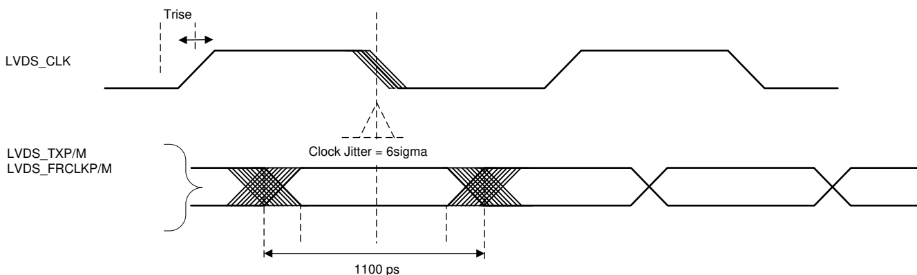
图 6-16. Timing Parameters
