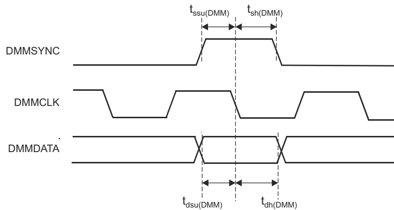
图 7-19. DMMDATA 时序
