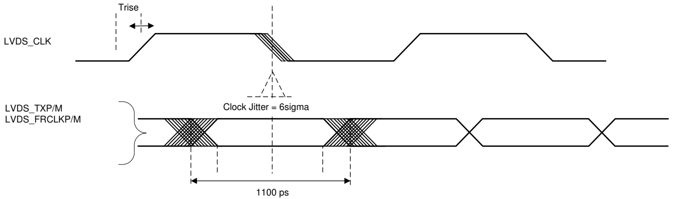
图 7-12. 计时参数
