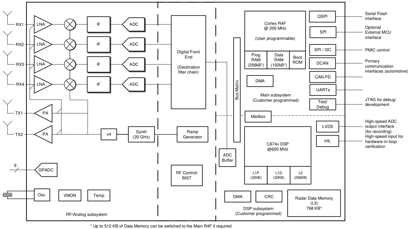
图 4-1. 功能方框图
