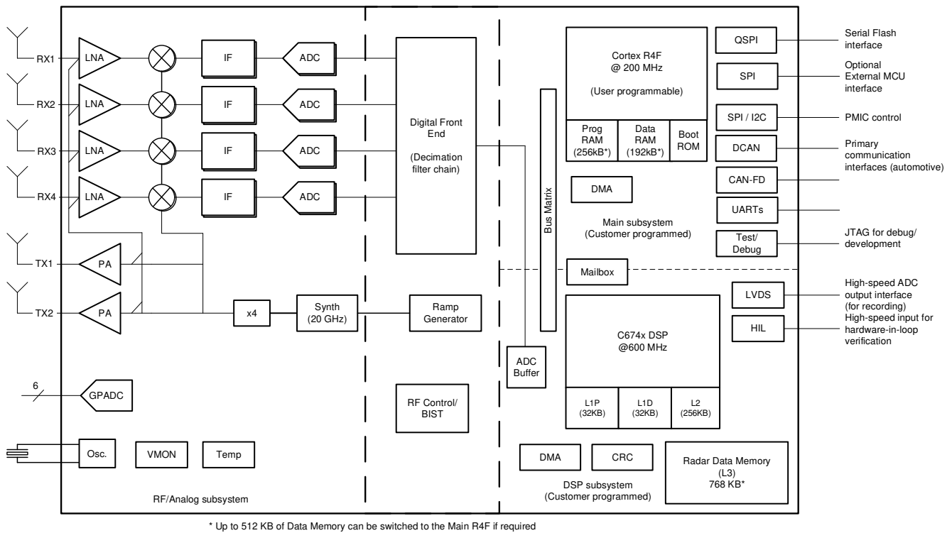
图 8-1. 功能方框图
