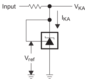
简化原理图
