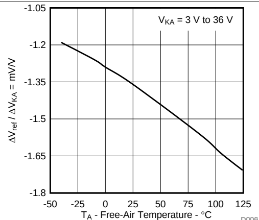
图 6. \Delta V_{ref} / \Delta V_{KA} 与自然通风温度间的关系
