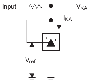
简化原理图
