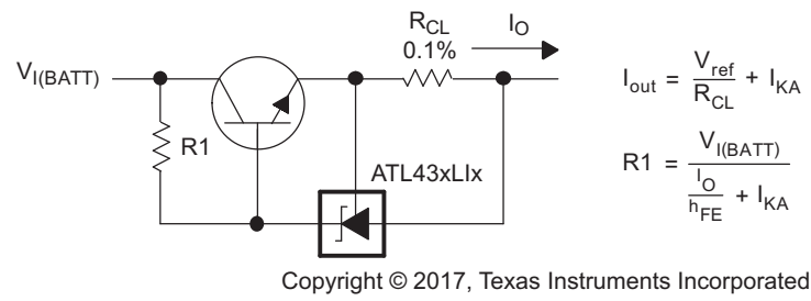
图 39. 精密限流器
