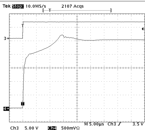
图 5-13. 脉冲响应
