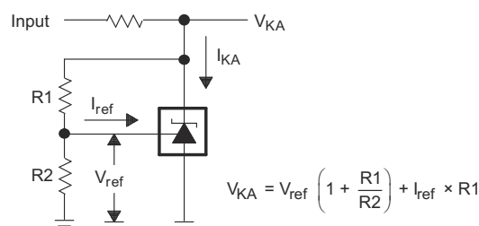
图 6-2. 针对 V_{\text{KA}} > V_{\text{ref}} 的测试电路
