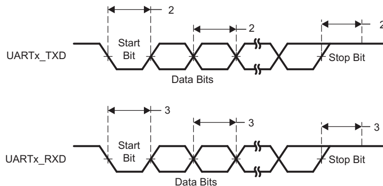
图 7-99. UART Timings
