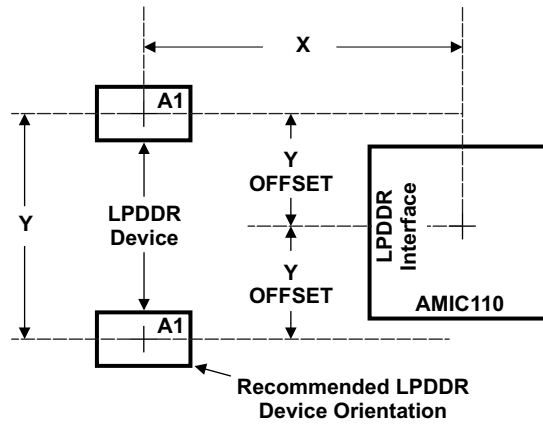
图 7-34. AMIC110 器件和 LPDDR 器件放置
