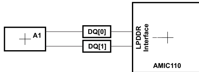
图 7-37. DQS[x] 和 DQ[x] 路由和拓扑
