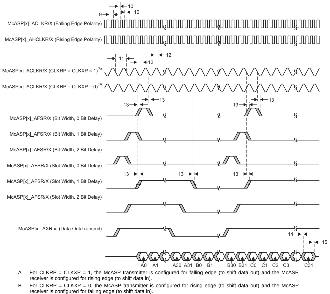
图 7-72. McASP Output Timing
