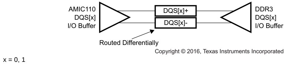
图 7-62. DQS[x] Topology
