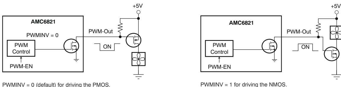
图 8-5. PWM Output
