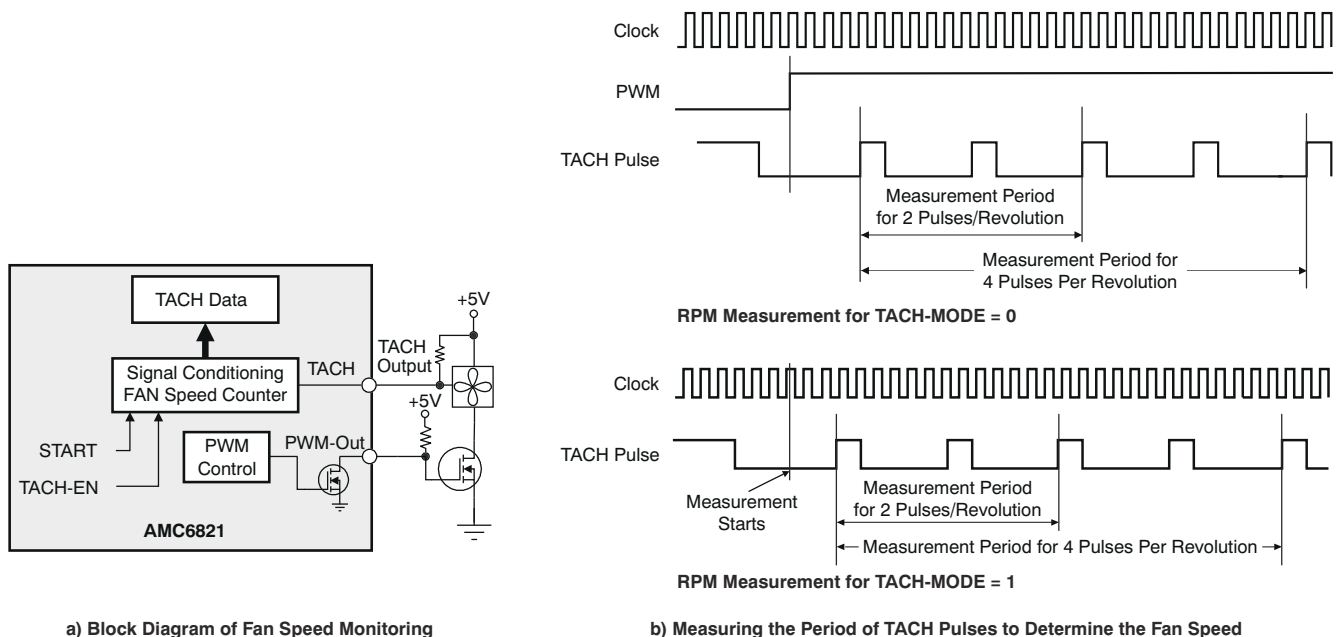
图 8-7. Fan Speed Measurement
