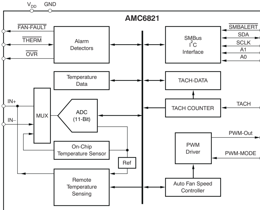
功能方框图
