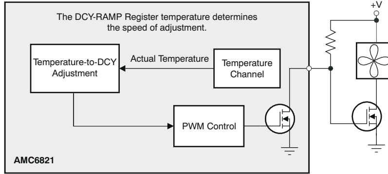
图 8-17. Auto Fan Temperature Loop
