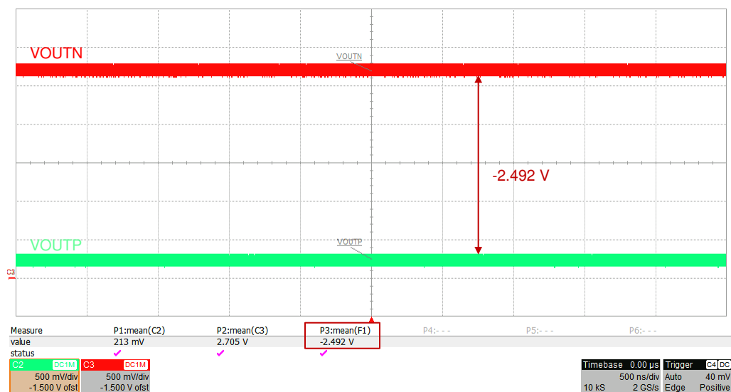
图 7-3. 典型的负差分输出：AMC3311
