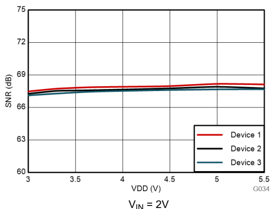
图 6-24. 信噪比与电源电压间的关系
