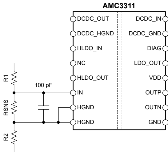
图 8-2. 输入滤波器
