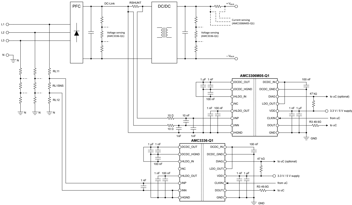
图 7-1. OBC 应用中的 AMC3306M05-Q1
