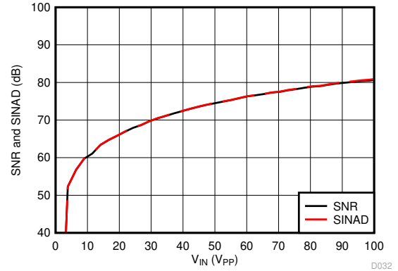
图 5-19. 信噪比和信纳比与输入信号幅度间的关系
