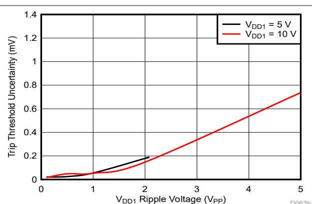
图 7-4. 跳变阈值对 VDD1 纹波电压的灵敏度 (Cmp1, f_{\text{RIPPLE}} = 10\text{kHz} )
