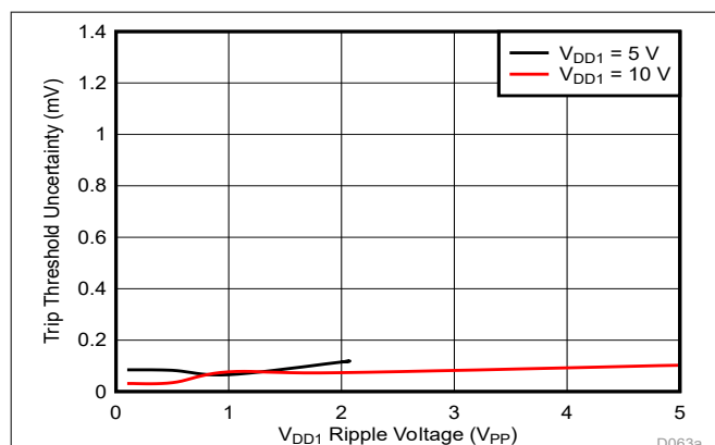
图 7-3. 跳变阈值对 VDD1 纹波电压的灵敏度 (Cmp0, f_{\text{RIPPLE}} = 10\text{kHz} )
