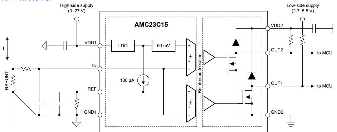
典型应用
