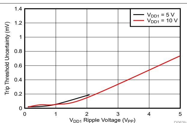
图 7-6. 跳变阈值对 V_{\text{DD1}} 纹波电压的灵敏度 (Cmp1, f_{\text{RIPPLE}} = 10\text{kHz} )
