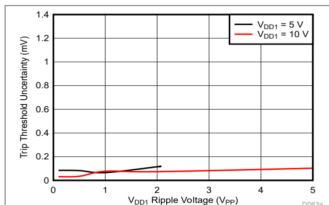
图 7-5. 跳变阈值对 V_{\text{DD1}} 纹波电压的灵敏度 (Cmp0, f_{\text{RIPPLE}} = 10\text{kHz} )
