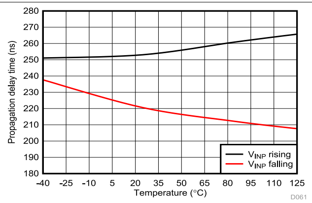
图 5-25. 传播延迟与温度间的关系
