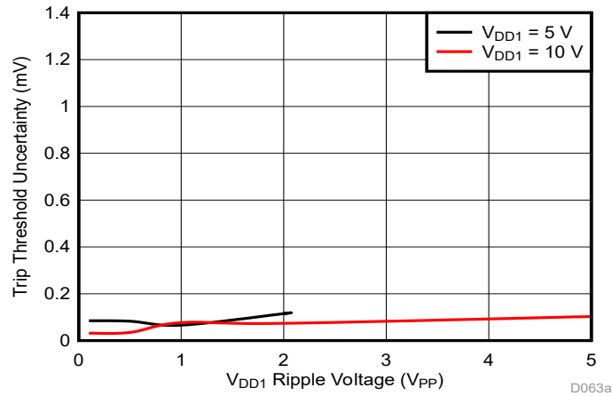
图 7-3. 跳变阈值对 VDD1 纹波电压的灵敏度 (f RIPPLE = 10KHz)
