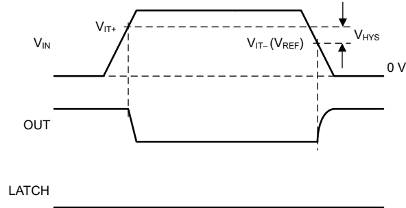
图 6-1. 开关阈值与迟滞
