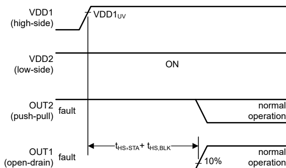
图 6-4. VDD2 保持开启; VDD1 开启 (长延迟)
