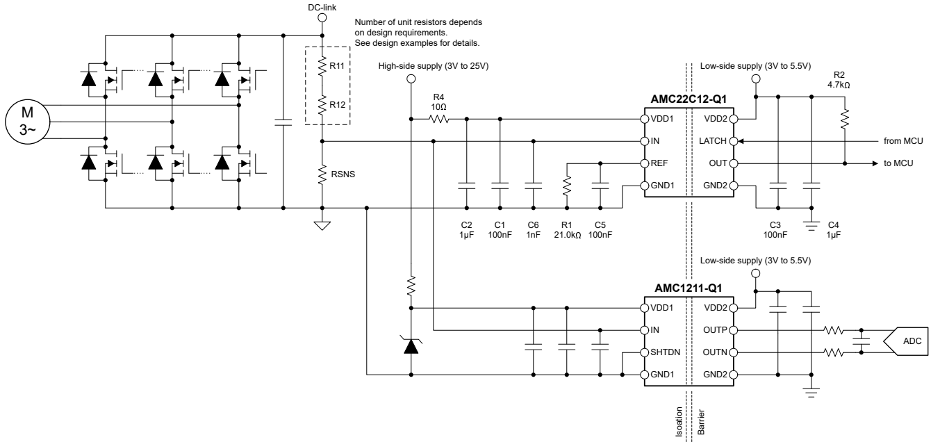
图 7-2. 使用 AMC22C12-Q1 进行过压检测
