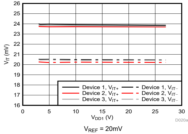
图 5-6. Cmp0 跳变阈值与电源电压间的关系
