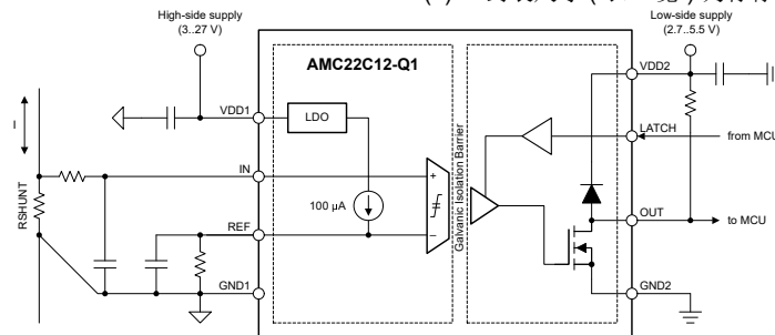
典型应用
