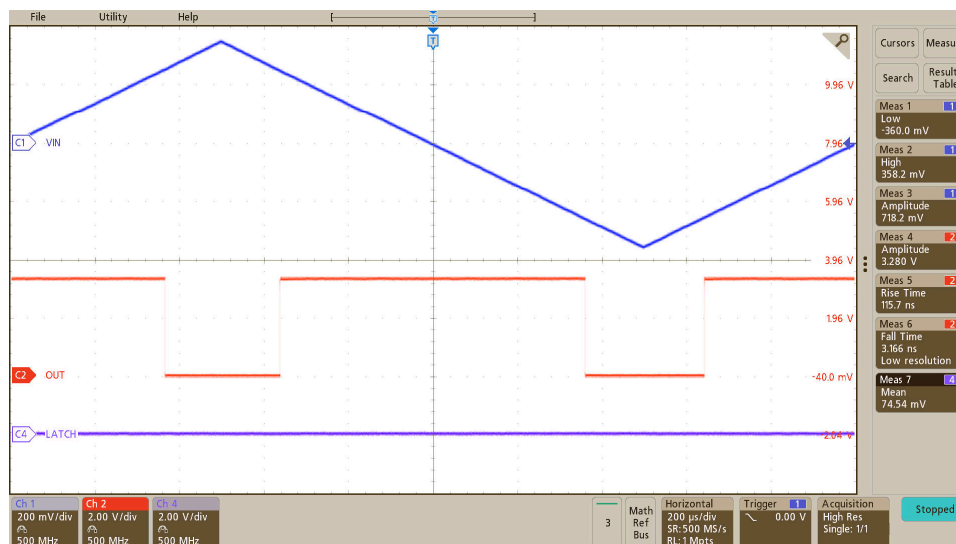
图 7-3. AMC22C12-Q1 对三角输入波形的输出响应
