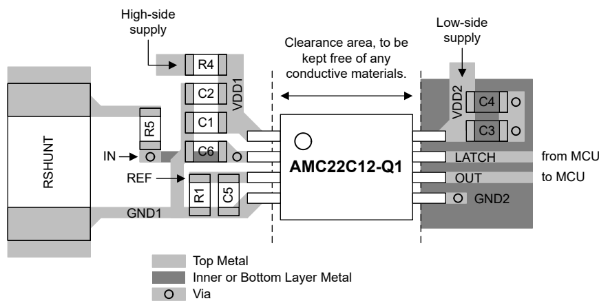
图 7-7. AMC22C12-Q1 的建议布局
