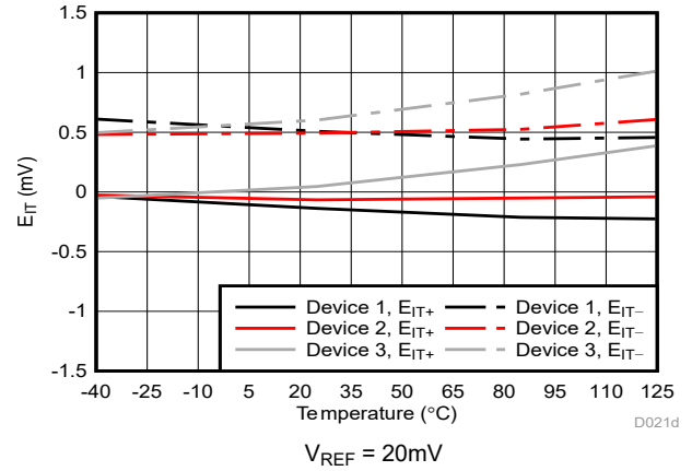
图 5-9. Cmp0 跳变阈值误差与温度间的关系
