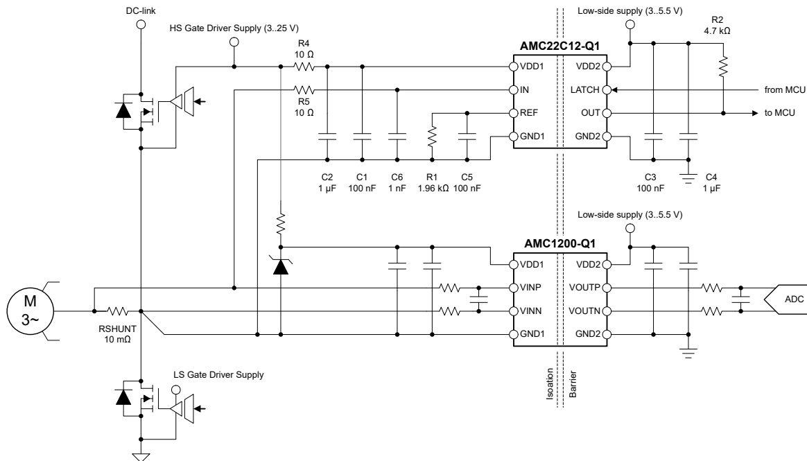
图 7-1. 使用 AMC22C12-Q1 进行过流检测
