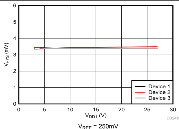
图 5-16. Cmp0 跳变阈值迟滞与电源电压间的关系
