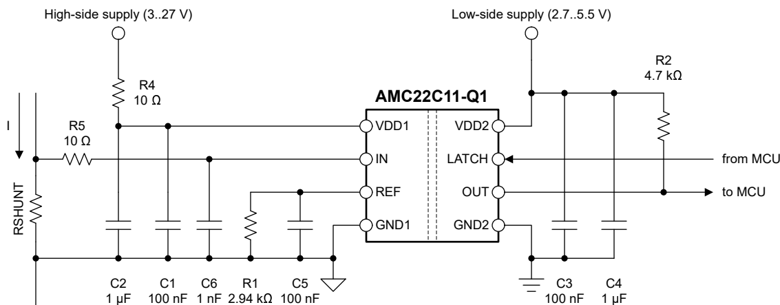
图 7-4. AMC22C11-Q1 去耦
