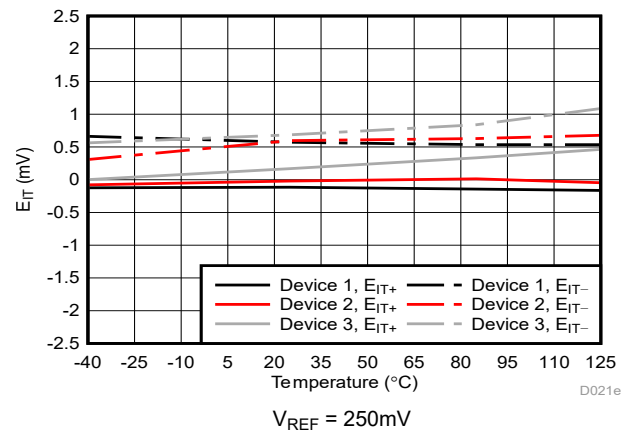
图 5-15. 跳变阈值误差与温度间的关系
