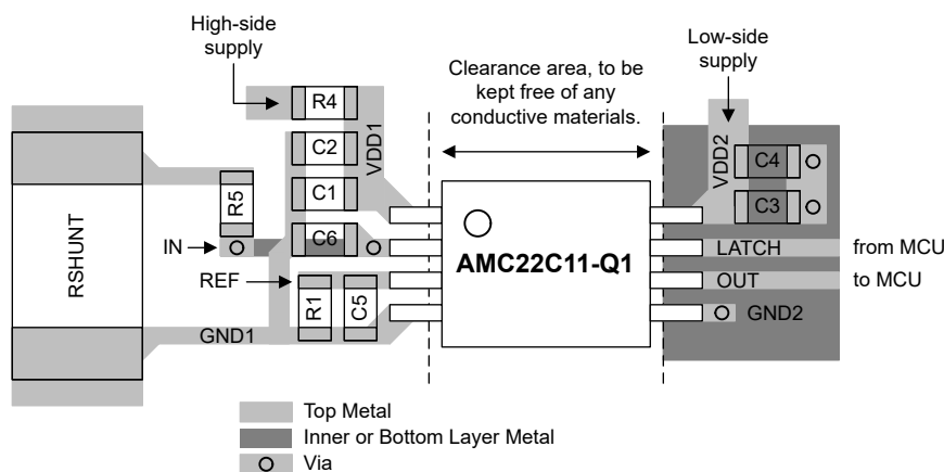
图 7-5. AMC22C11-Q1 的建议布局
