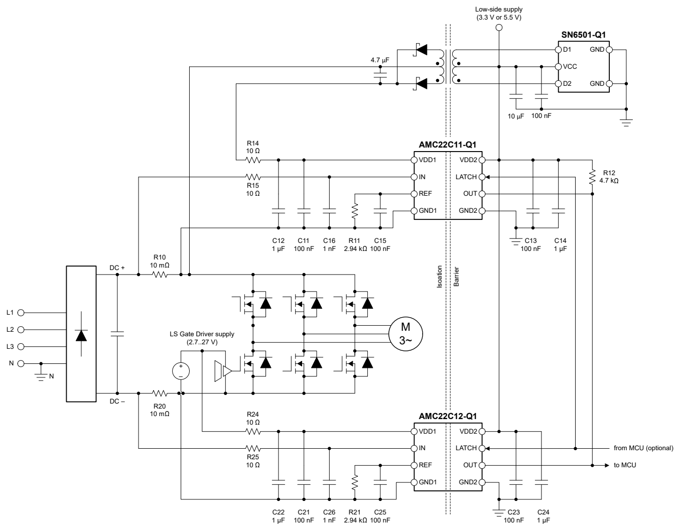
图 7-1. 使用 AMC22C11-Q1 进行 DC+ 过流检测
