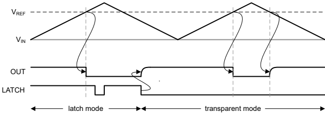
图 5-2. 功能时序图
