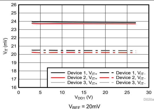
图 5-6. 跳变阈值与电源电压间的关系
