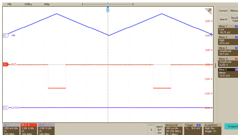
图 7-2. AMC22C11-Q1 对三角输入波形的输出响应
