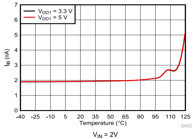
图 5-27. 输入偏置电流与温度间的关系
