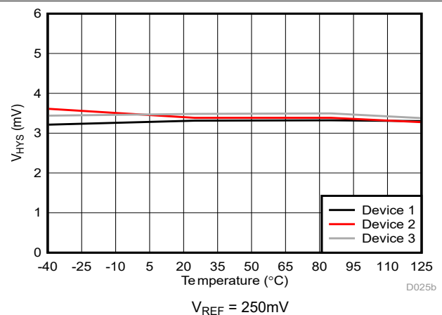
图 5-17. 跳变阈值迟滞与温度间的关系
