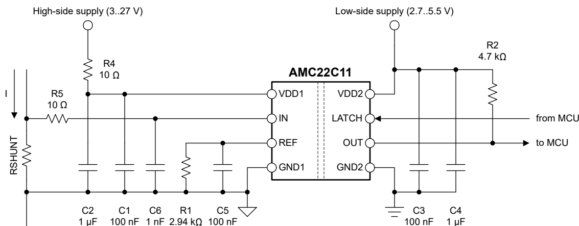
图 7-4. AMC22C11 去耦
