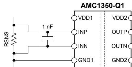
图 8-2. Input Filter
