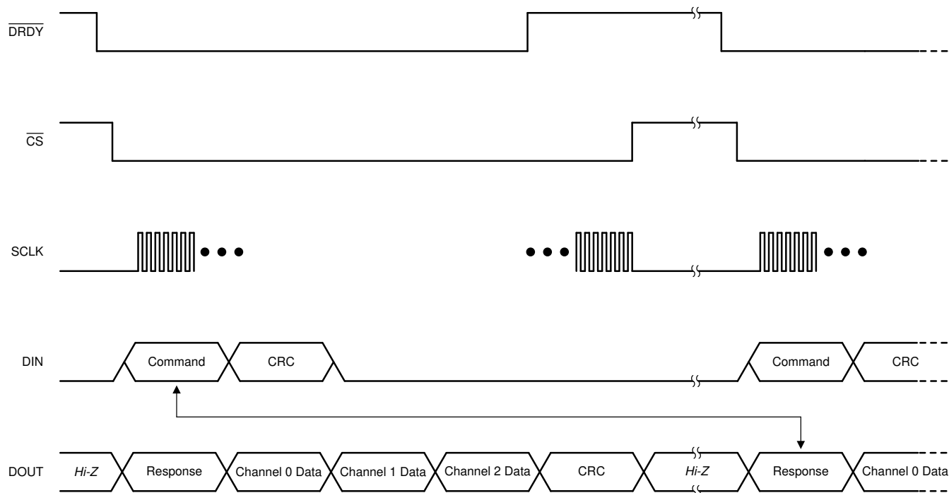
图 8-24. 典型通信帧
