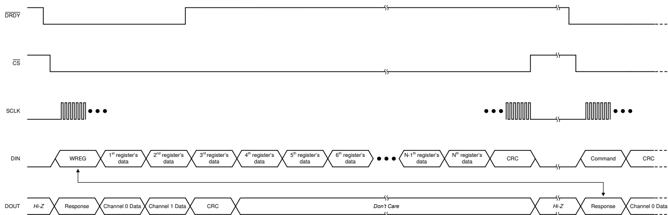
图 8-27. 写入寄存器
