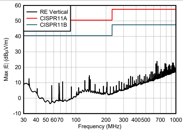
图 9-7. AMC130M03 垂直辐射发射 CISPR11 测量
