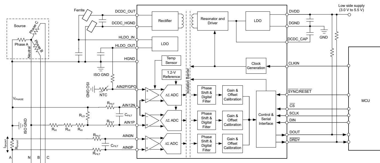
图 9-5. 电流和电压检测 - 使用 AMC130M03
