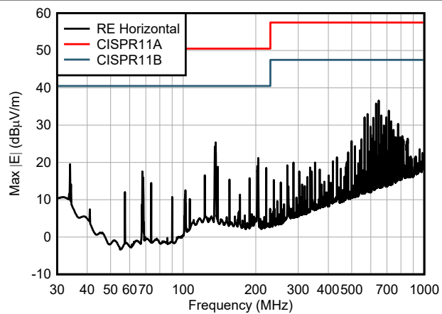
图 9-6. AMC130M03 水平辐射发射 CISPR11 测量
