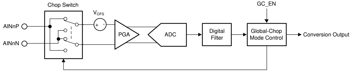
图 8-20. 全局斩波模式实现
