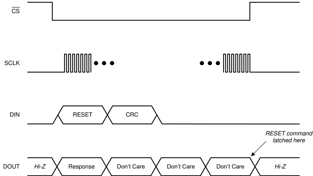
图 8-24. RESET 命令帧
