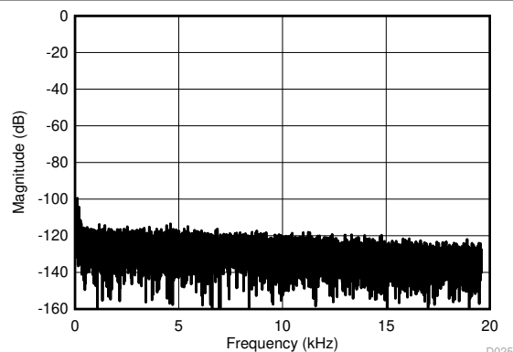
图 6-31. 35Hz 输入信号时的频谱
