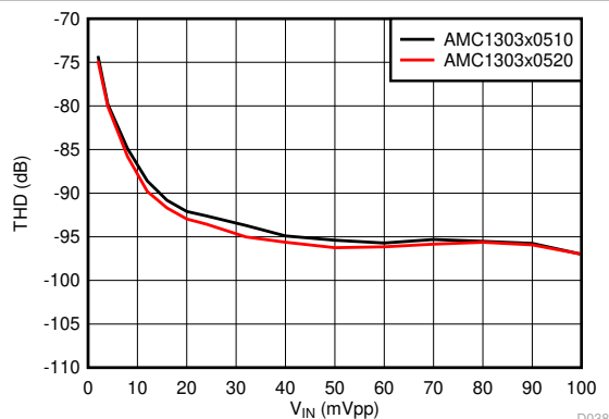
图 6-25. 总谐波失真与输入信号幅度间的关系
