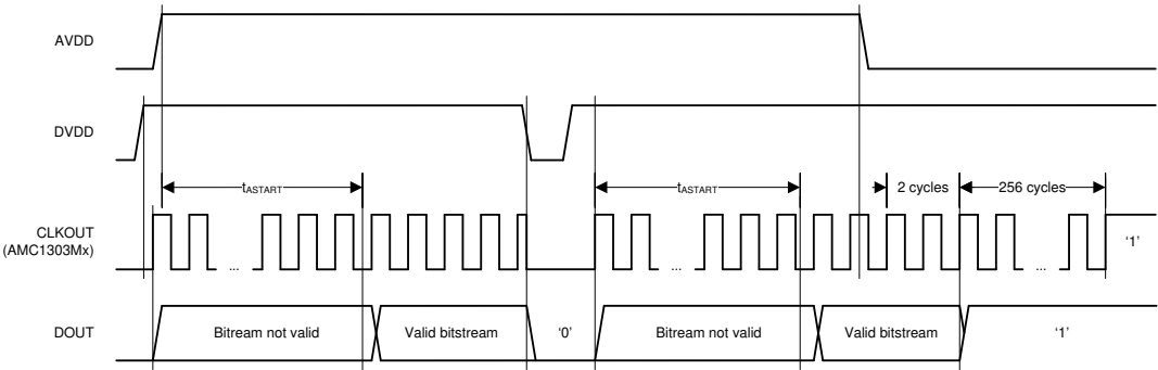
图 6-2. 数字接口启动时序
