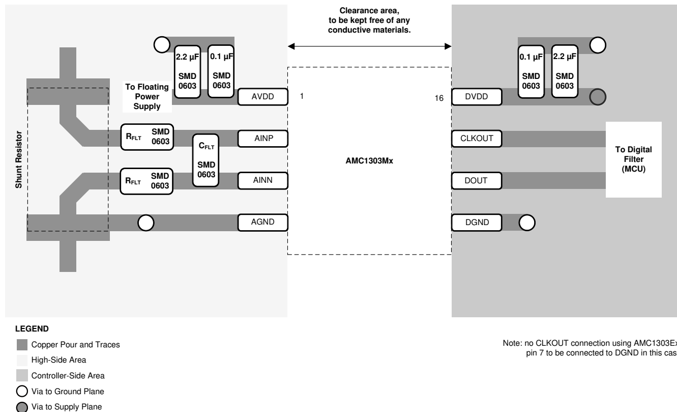
图 8-9. AMC1303 的建议布局
