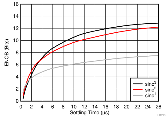
图 8-5. 测得的有效位数与建立时间间的关系
