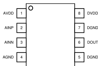
图 5-2. AMC1303Ex : DWV 封装 , 8 引脚 SOIC ( 顶视图 )
