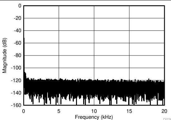
图 6-32. 35Hz 输入信号时的频谱
