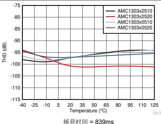
图 6-22. 总谐波失真与温度间的关系
