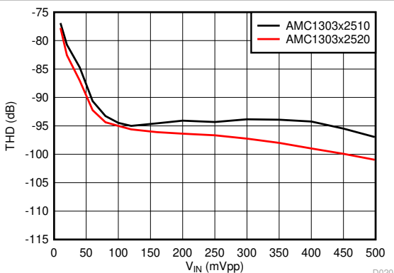
图 6-24. 总谐波失真与输入信号幅度间的关系
