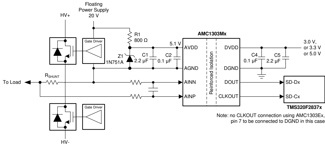
图 8-8. 对 AMC1303 去耦
