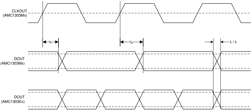
图 6-1. AMC1303Mx 数字接口时序
