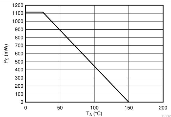
图 6-4. 安全限制功率的热降额曲线 (符合 VDE)
