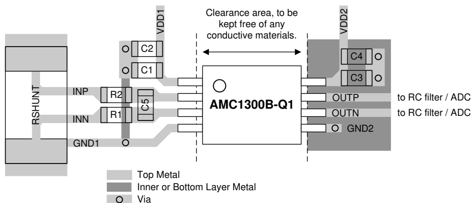
图 10-1. Recommended Layout of the AMC1300B-Q1
