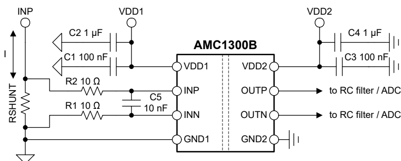
图 10-1. Decoupling of the AMC1300
