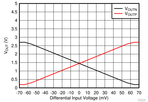
图 6-18. Output Voltage vs Input Voltage
